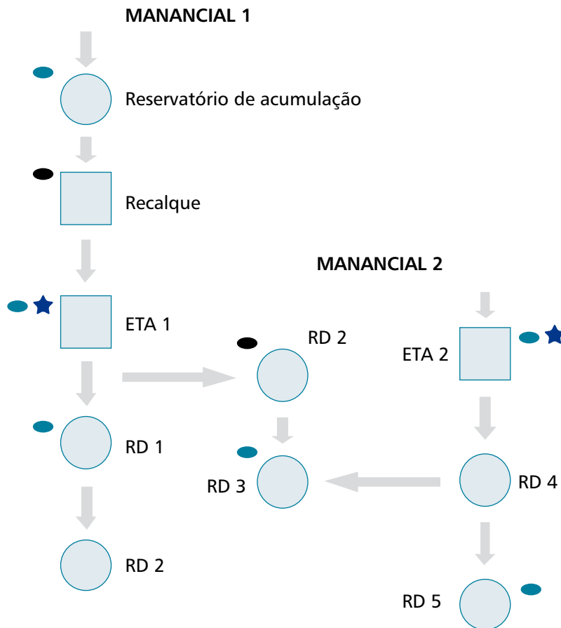
Figura 3. Exemplo de diagrama de fluxo de sistema de abastecimento de água.
