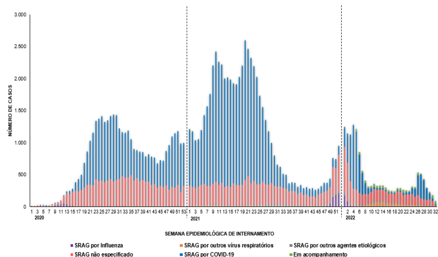
Figura 6. Casos de Síndrome Respiratória Aguda Grave Hospitalizados, segundo classificação final do caso e semana epidemiológica de internamento, SE 01 de 2020 a SE 32 de 2022. Bahia, 2020-2022.
