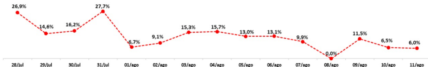
Figura 8. Proporção de resultados positivos para SARS CoV-2 liberados/dia. Bahia, produção LACEN/BA - Julho/Agosto 2022.
